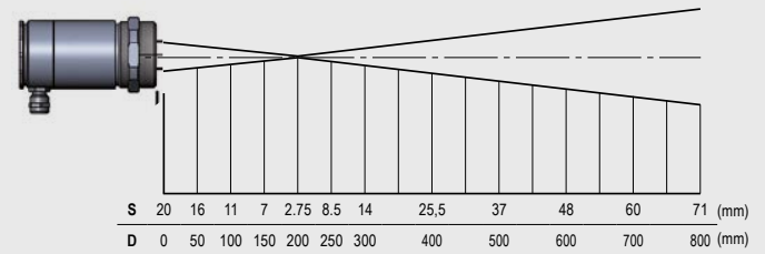
CF3 optics 75:1
